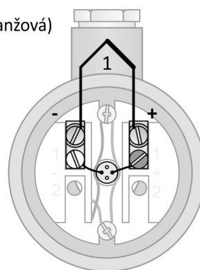
Obrázek 1.5: zapojení jednoduchého termočlánu
