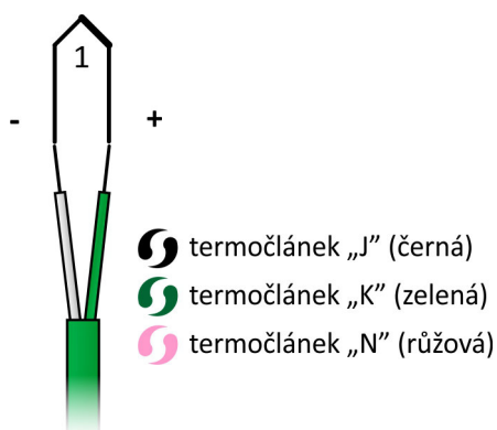
Obrázek 11U.7: Zapojení jednoduchého termočláčku
