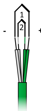
Obrázek 11U.8: Zapojení dvojitého termočláčku
