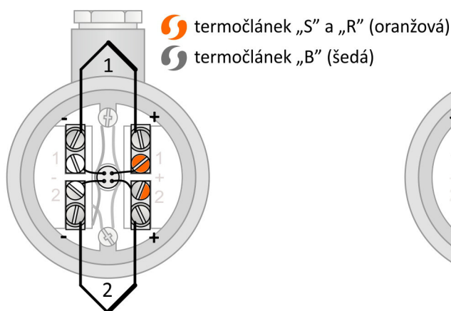
Obrázek 2L.4: zapojení dvojitého termočláčku
