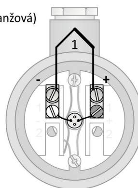
Obrázek 2L.5: zapojení jednoduchého termočláčku
