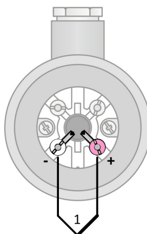
Obrázek 6M.8: zapojení jednoduchého termočlánu
