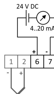
Obrázek 6MA.8: zapojení převodníku
