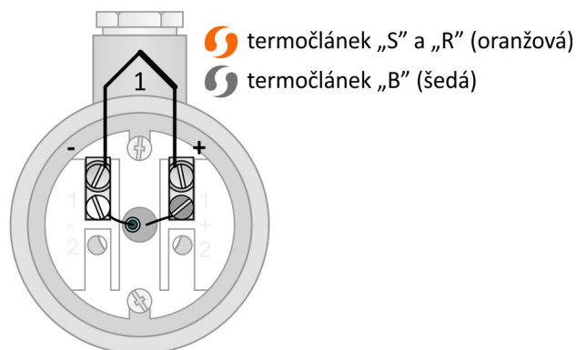
Obrázek 6S.3: zapojení jednoduchého termočláneku
